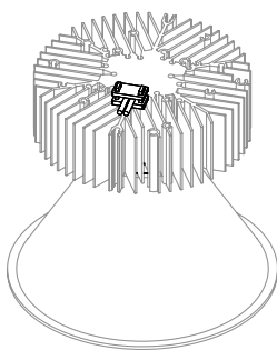
Kábelrögzítő/Cable lock
